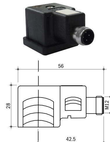
Adattatore DIN 43650 A a M12 DIN 43650 A to M12 adaptor
