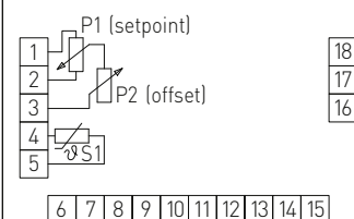
Aansluitschema RTFxx P
